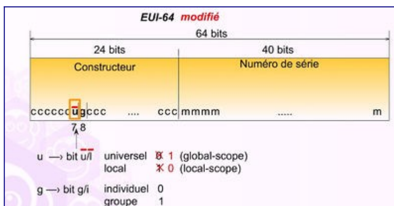
Figure 8 : Identifiant d'interface dérivé du format EUI-64.
