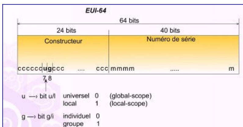
Figure 7 : Format de l'identificateur IEEE EUI-64.
