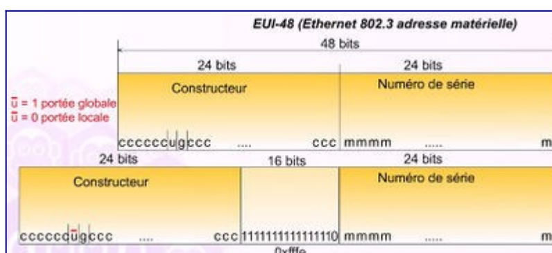
Figure 9 : Identifiant d'interface dérivé de l'adresse MAC (EUI-48).
